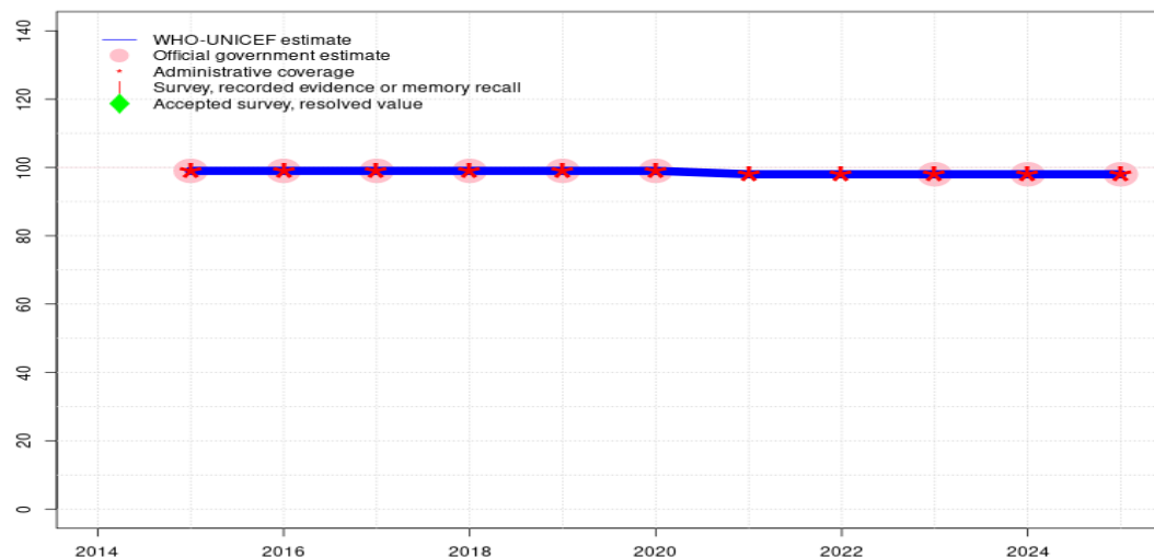
ALB - IPV1
