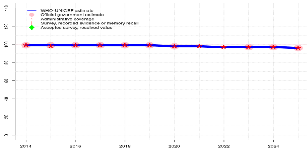
ALB - DTP3
