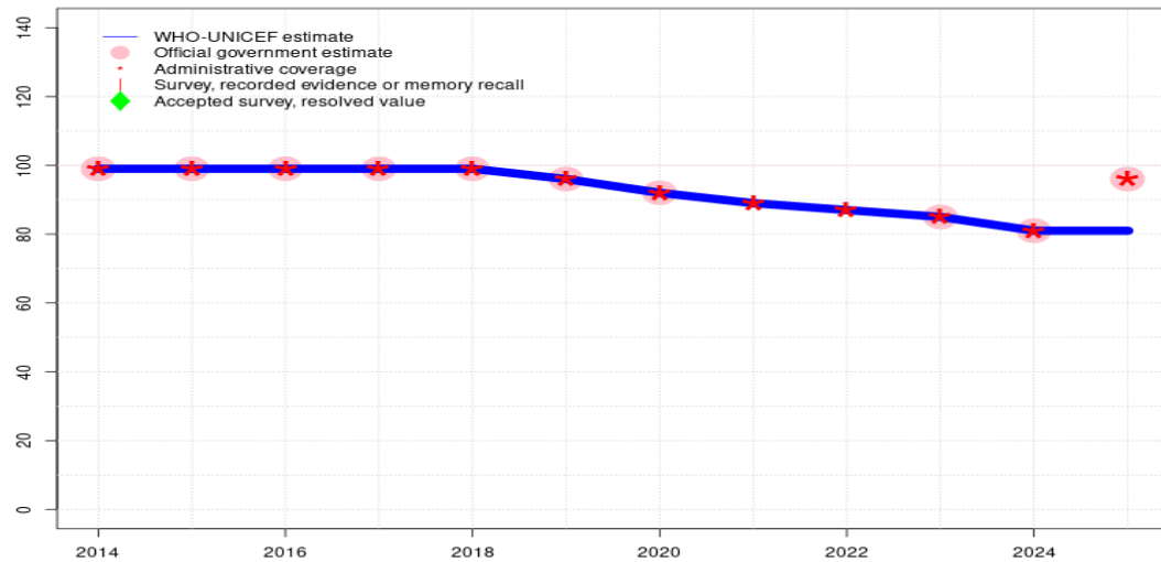
ALB - PCVC
