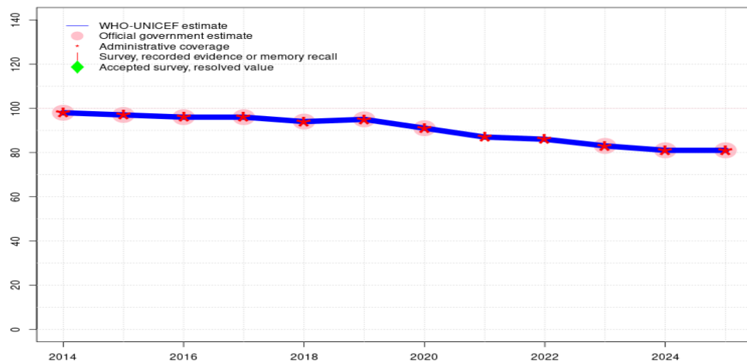
ALB - MCV1
